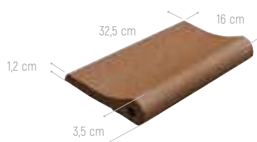
BORDE PISCINA 16 16 x 32,5 cm - 6.3"x 12.8"
