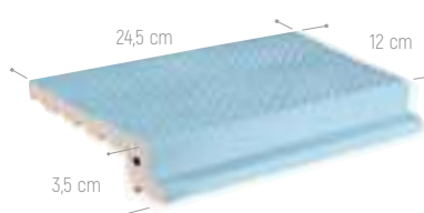
REF. 919 SOPORTE REJILLA SPORT 13,5 x 24,5 x 3,5 cm - 5.3"x 9.6"x1.4"
