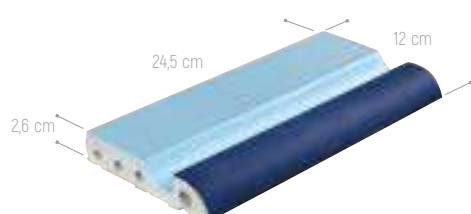
REF. 953 BORDE FINLANDÉS 12 x 24,5 x 2,6 cm - 4.7"x 9.6"x1.0"
