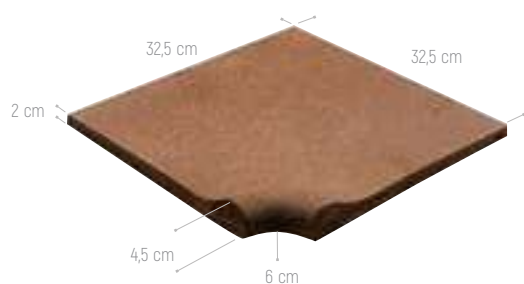
ESQUINA INTERIOR 33 32,5 x 32,5 cm - 12.8"x 12.8"
