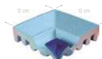
REF. 313 ÁNGULO INT. FINLANDÉS 12 x 12 cm - 4.7"x 4.7"
