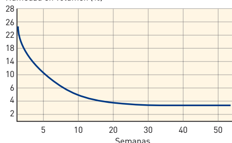
Curva de secado de los bloques de hormigón celular YTONG de 20 cm de espesor en temperatura ambiente interior
