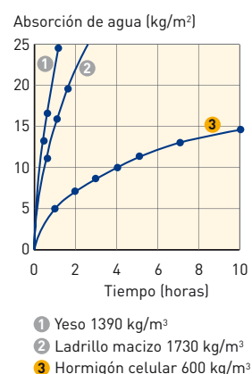
Absorción de agua de diferentes materiales
