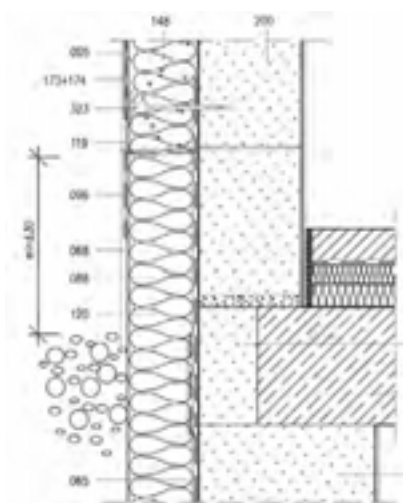
Perfil de zócalo
