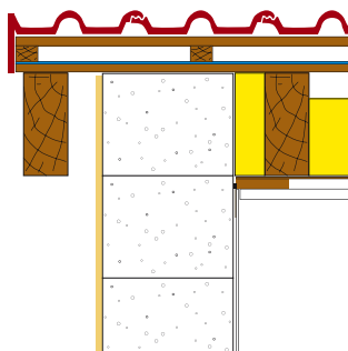
Variante muro YTONG
