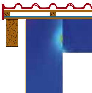
Variante hormigón celular
