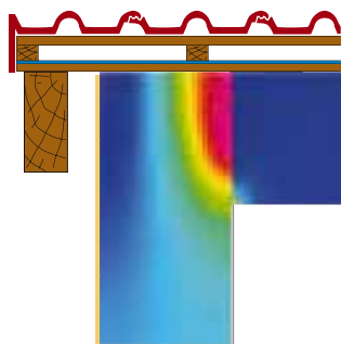
Variante ladrillo perforado
