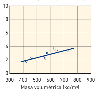
Proporción de humedad de equilibrio (en volumen) en función de la masa volumétrica
