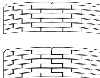
Plano de rotura perpendicular a los tendeles (flexión horizontal)
