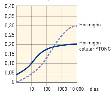
Retracción en mm/m
