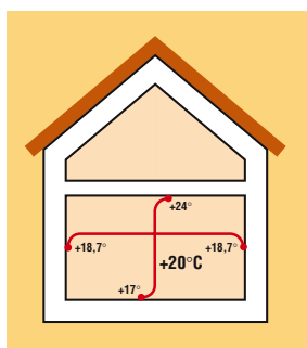
Confort térmico en el interior de una vivienda construida en hormigón celular
