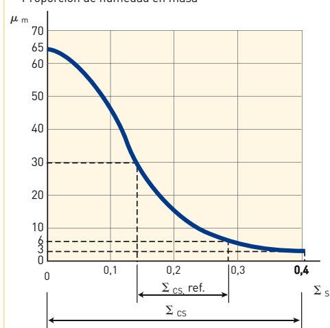
Retracción en mm/m
